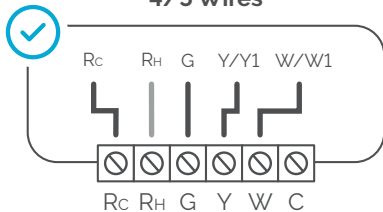
4/5 Wires
